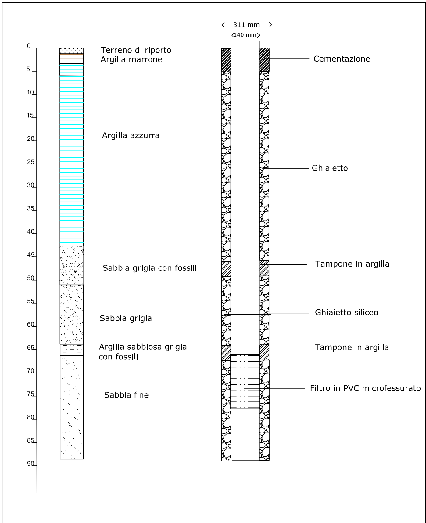
Stratigrafia e Schema costruttivo pozzo AGBALT
